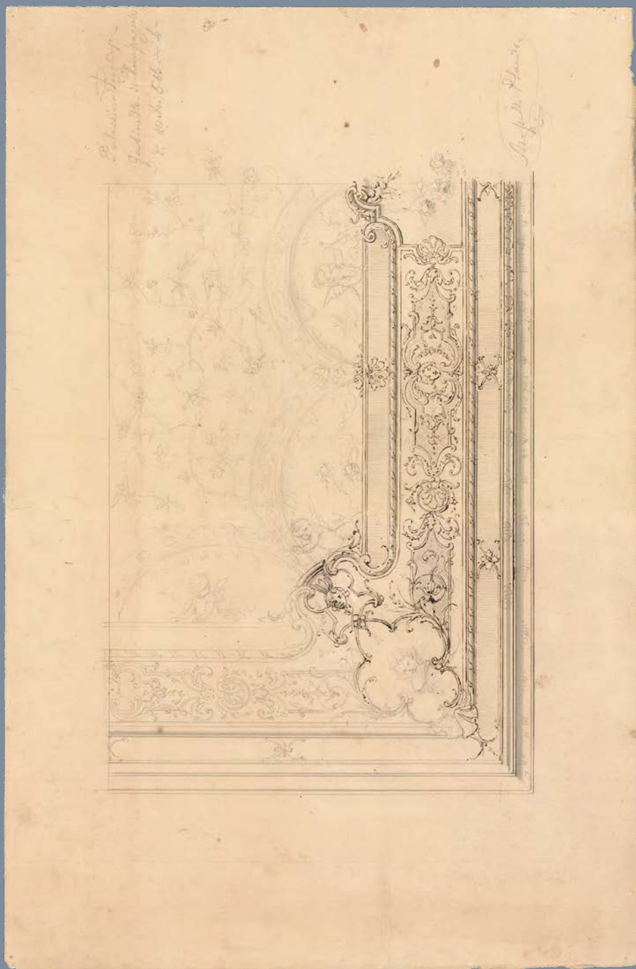
Placido Mosello, Palazzina Pugliese . Gabinetto di compagnia di metri 5,65 x 4, s.d. (MC_695).
